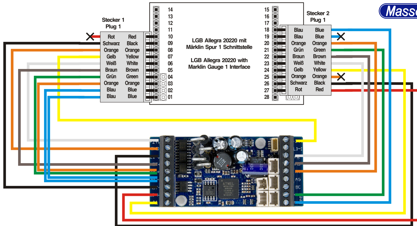
Schematische Darstellung Anschluss XLS an Spur 1 Schnittstelle von Märklin. Üblicherweise sollten die Stecker von der Innenseite an der Schnittstelle angeschlossen werden (hier zur Verdeutlichung von außen). Schematic illustration of XLS installation with Märklin Gauge 1 Interface. Usually the plugs should connect from the interior side of the interface (illustration shows connection from outside). Irrtümer und Änderungen vorbehalten. Errors and omissions accepted.
